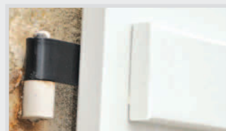
PLIAGE DES PENTURES : adaptation aux gonds existants
