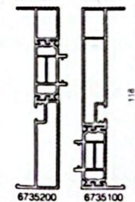
Montants dormants monobloc sans rails
