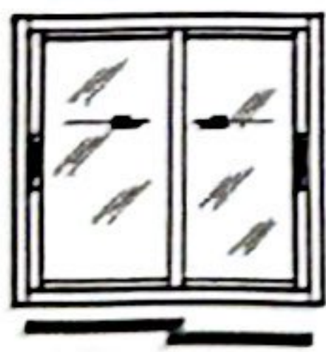
Coulissant bi-rails 2 à 4 vantaux Coupe droite et coupe d'onglet
